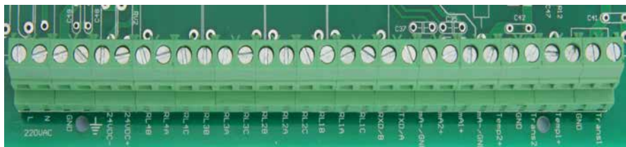
◆水下测距仪接线端子示意图
