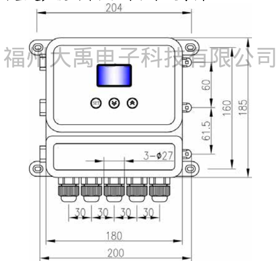
分体型超声波测深仪
