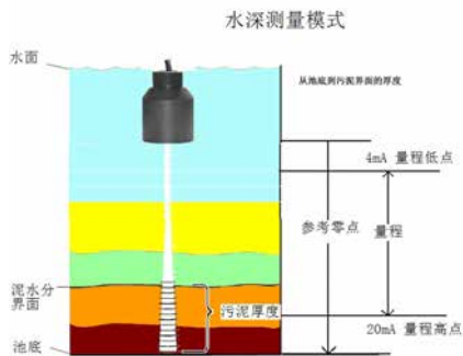
附图 1.1 水深测量示意图
